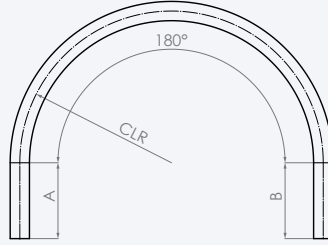
180° Long Radius Bend
