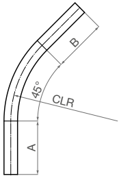
45° Long Radius Bend
