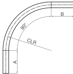
90° Long Radius Bend
