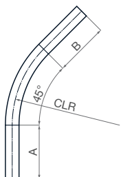
45° Long Radius Bend
