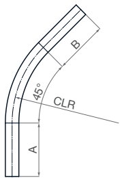
45° Long Radius Bend
